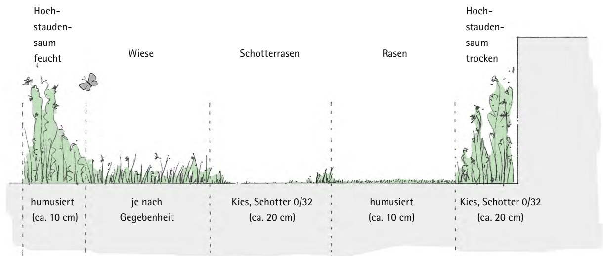
Abb. 12: Bodenaufbau von Rasen, Schotterrassen, Wiese und Hochstaudensaum.
