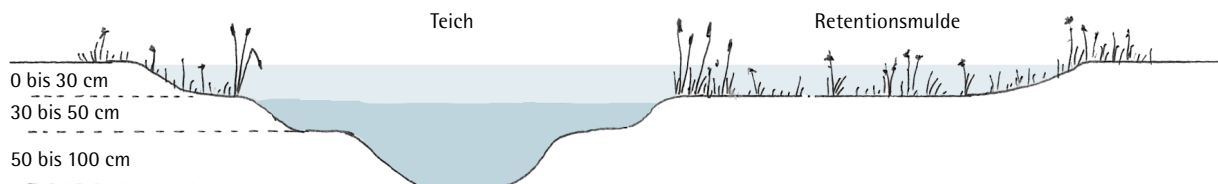
Abb. 14: Neuanlage von (Klein-)Gewässern mit Retentionszone.
